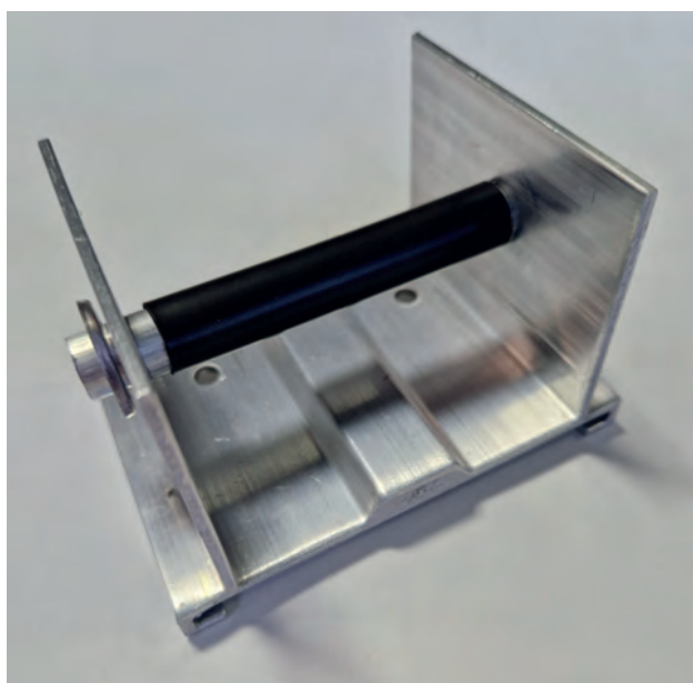
Profilo Omega e Rondello allaccio per facciate.
