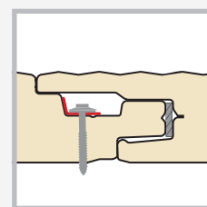
Particolare - Fissaggio nascosto Uni Wall
